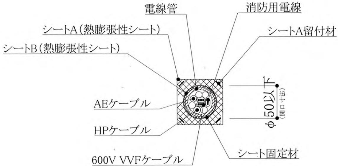
立面図
